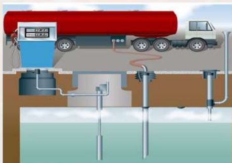
Compteur volumétrique pour station à essence
